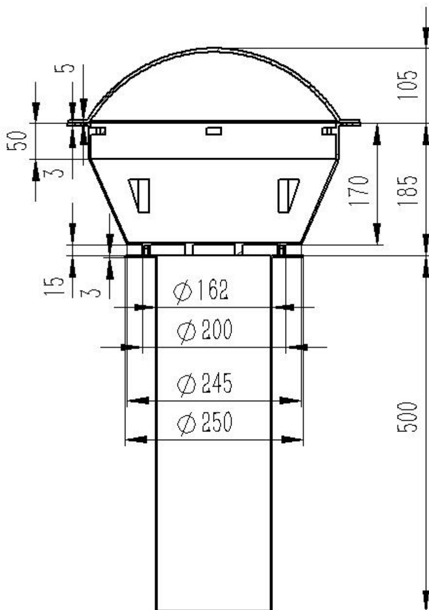
图 7：浮标体尺寸图
